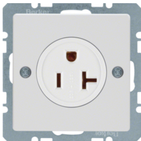
Zásuvka s ochranným kontaktem, USA / KANADA NEMA 5-20 R, Q.x, bílá sametová
